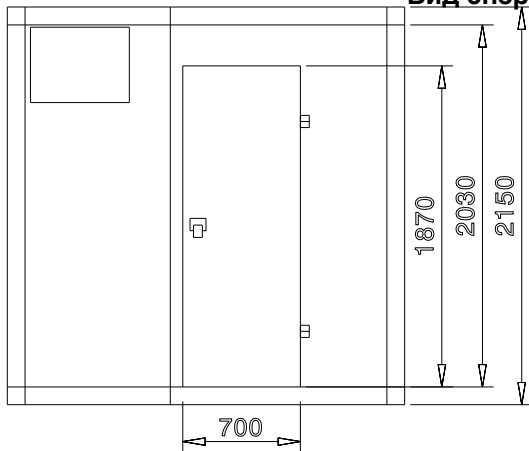
Вид сбоку
