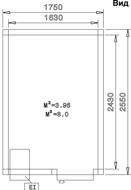
Вид сверху
