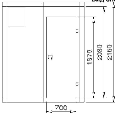
Вид сбоку
