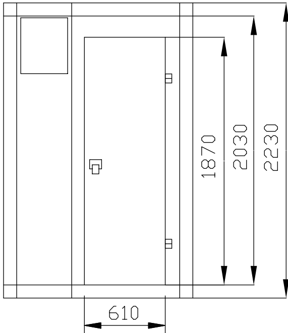
Вид спереди
