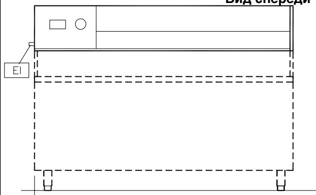
Вид сбоку
