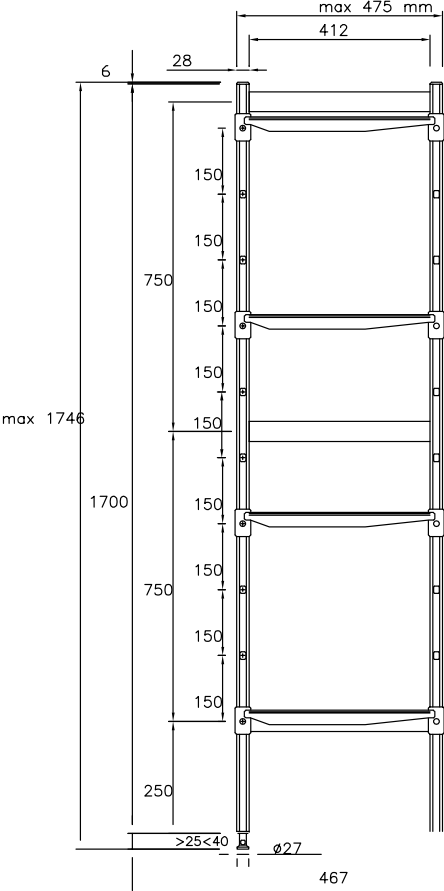
Вид спереди
