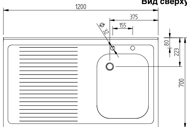
Вид сверху
