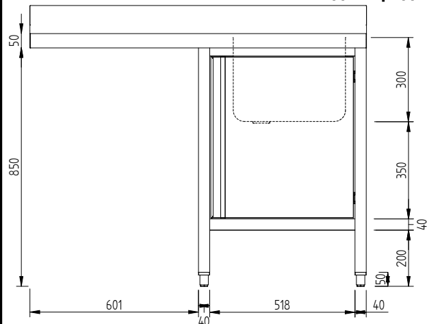
Вид спереди
