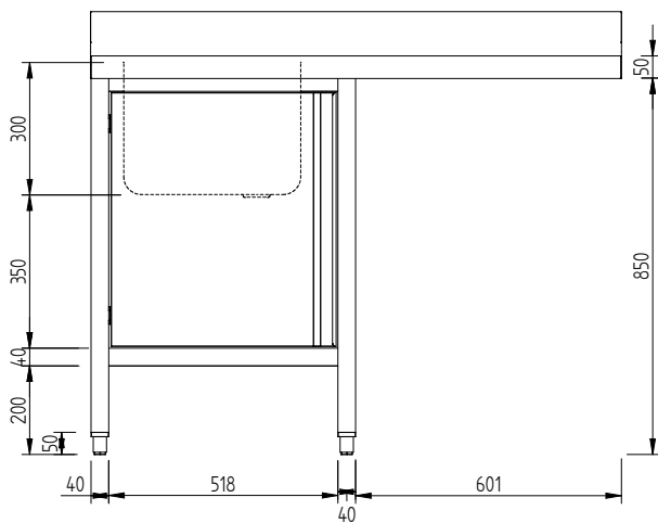
Вид сбоку
