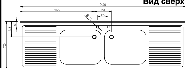
Вид сверху
