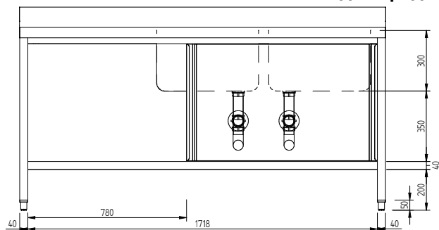
Вид спереди
