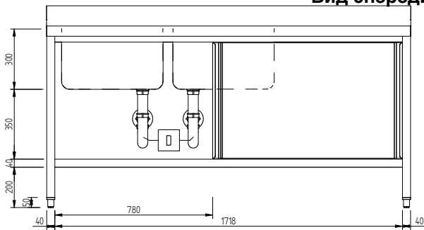
Вид сбоку
