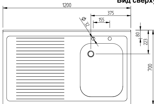
Вид сверху
