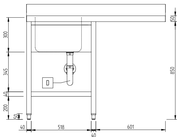
Вид сбоку
