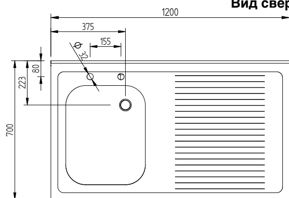
Вид сверху
