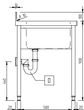
Вид сбоку
