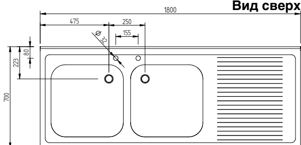
Вид сверху
