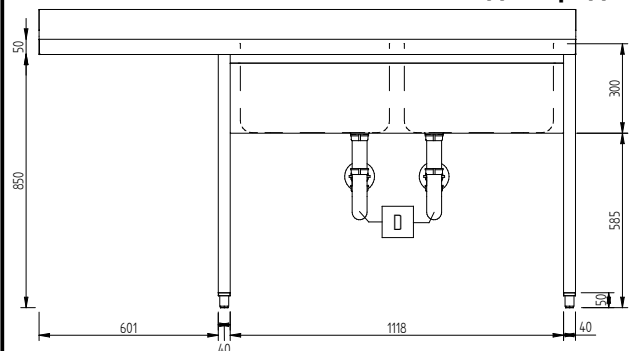
Вид спереди
