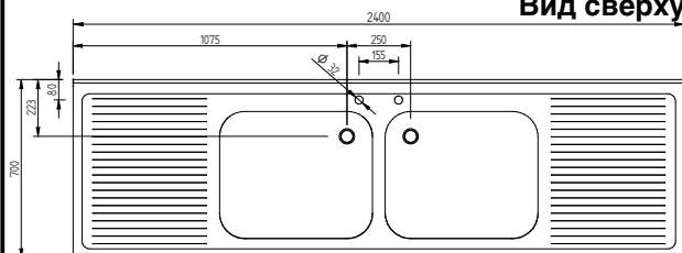
Вид сверху
