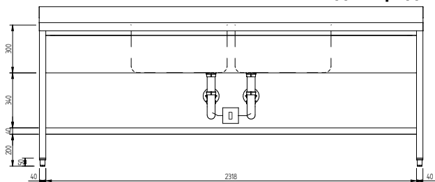
Вид спереди
