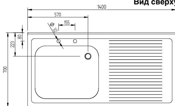
Вид сверху
