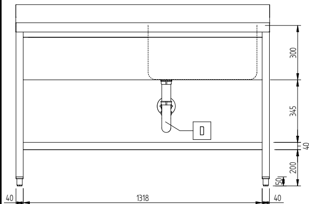
Вид спереди
