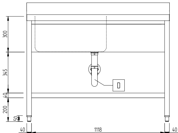
Вид спереди
