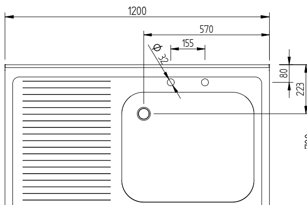
Вид сверху
