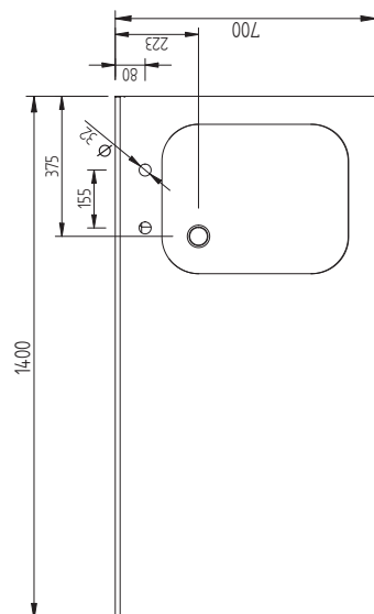
Вид сверху
