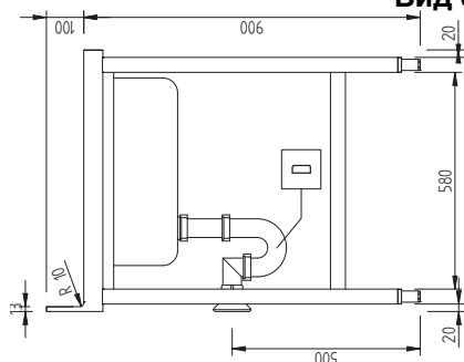
Вид спереди
