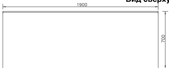
Вид сверху
