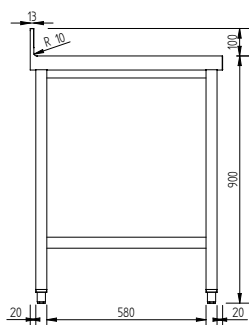
Вид сбоку
