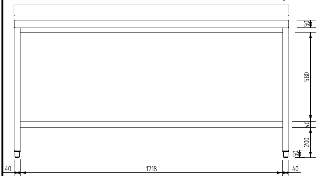
Вид спереди
