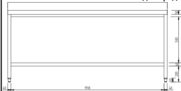
Вид спереди
