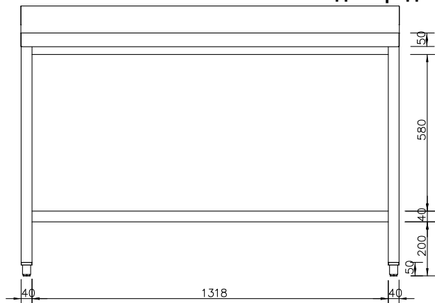
Вид спереди
