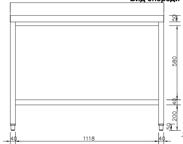
Вид сбоку
