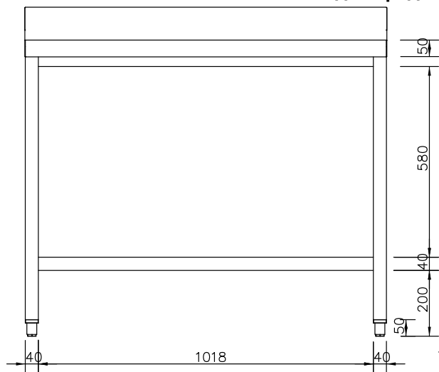
Вид спереди
