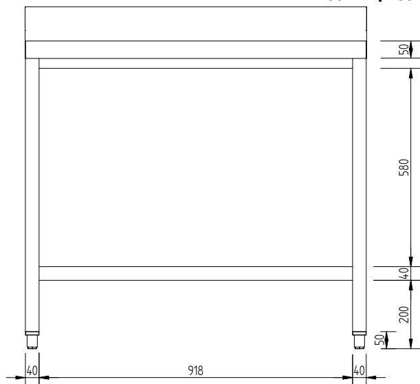
Вид спереди
