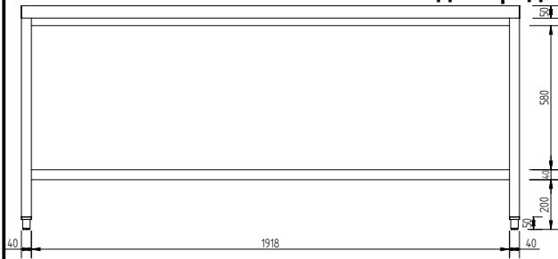
Вид сбоку
