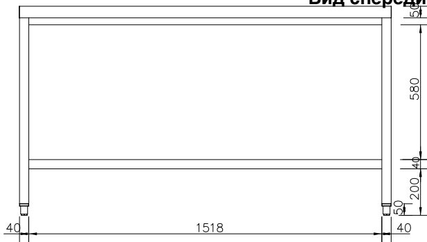
Вид сбоку
