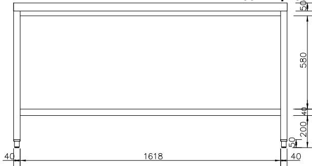
Вид спереди
