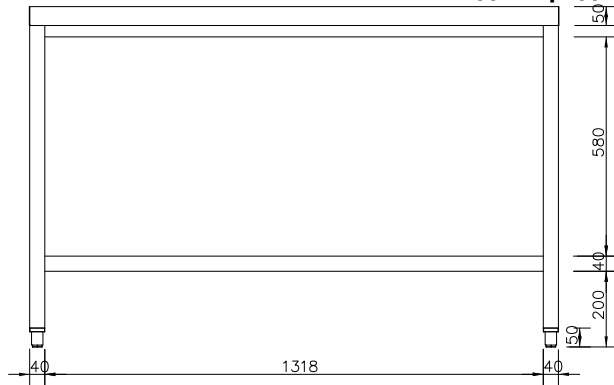
Вид сбоку
