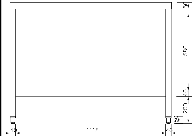
Вид спереди
