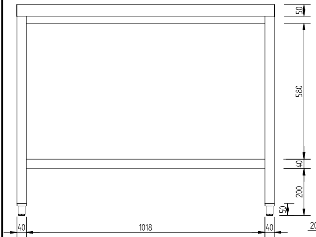
Вид спереди
