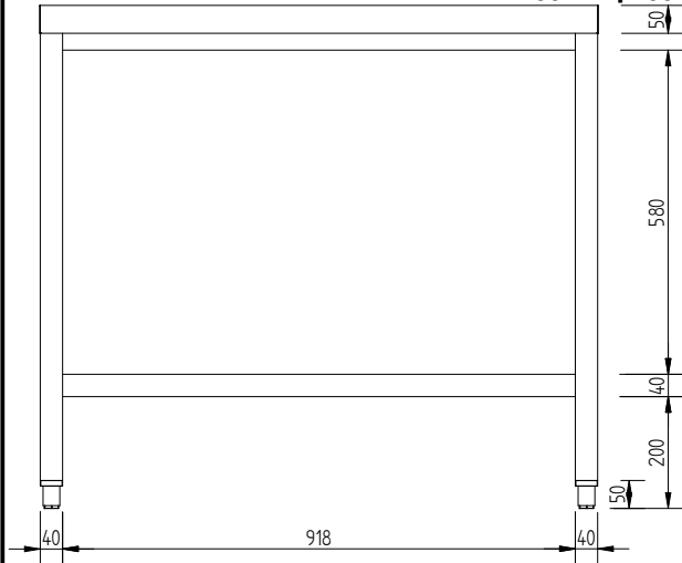
Вид спереди
