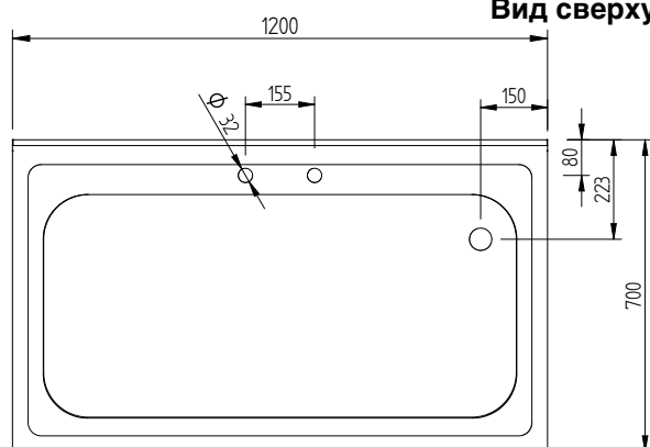
Вид сверху
