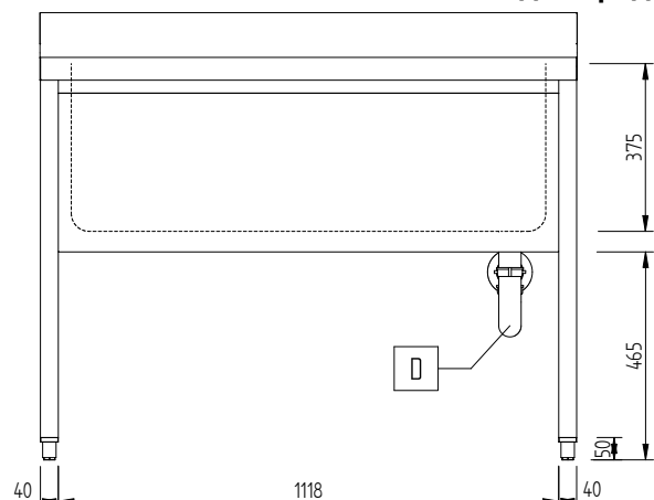
Вид спереди
