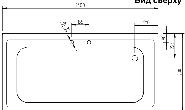
Вид сверху
