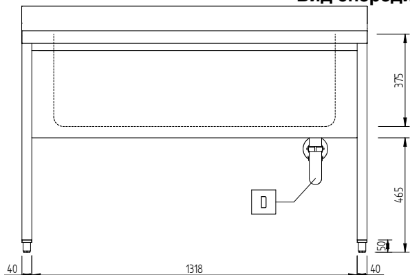
Вид сбоку
