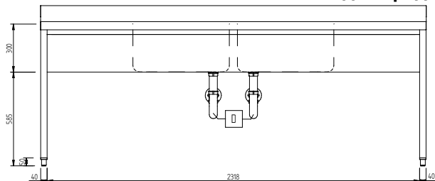
Вид спереди
