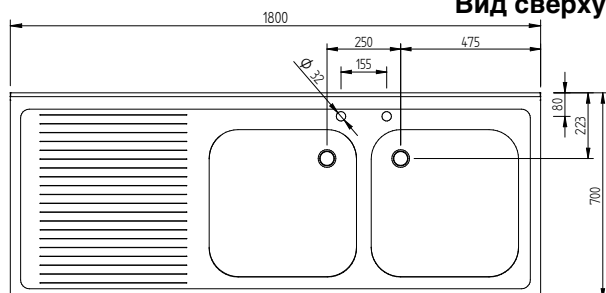
Вид сверху
