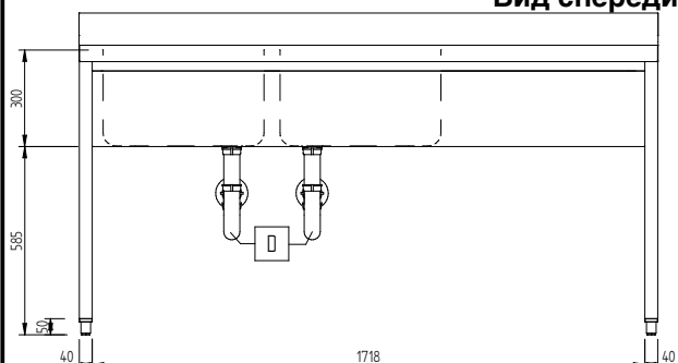
Вид спереди
