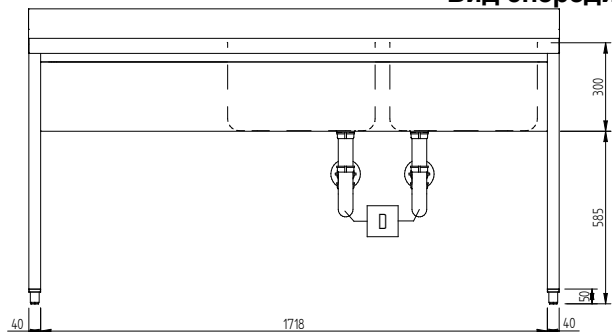
Вид сбоку
