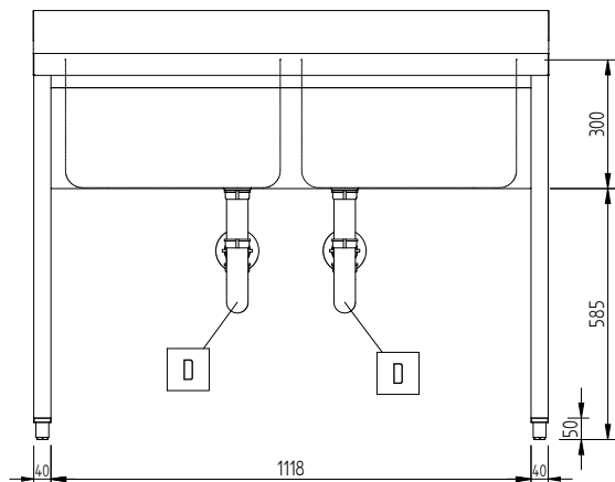
Вид сбоку
