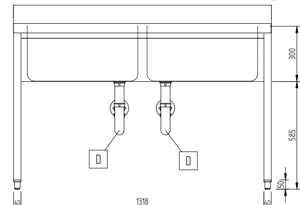
Вид спереди
