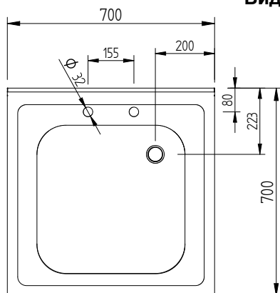
Вид сверху
