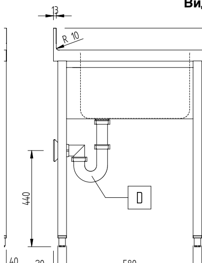
Вид сбоку
