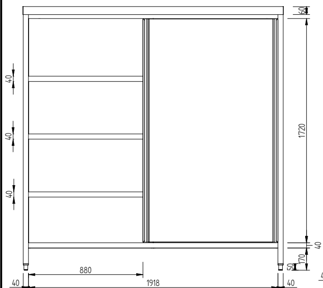
Вид спереди
