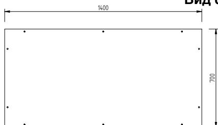
Вид сверху
