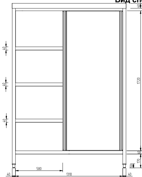
Вид сбоку
