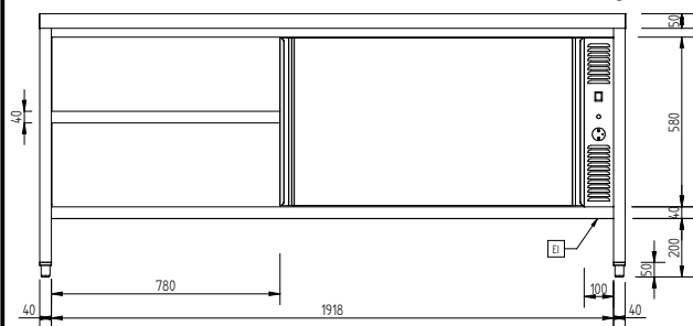
Вид спереди
