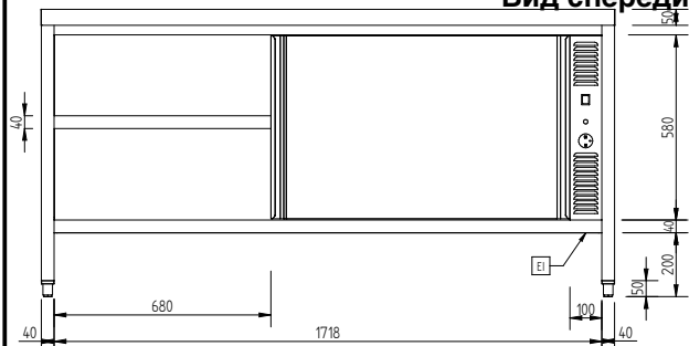
Вид спереди
