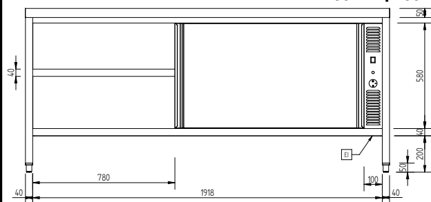
Вид спереди
