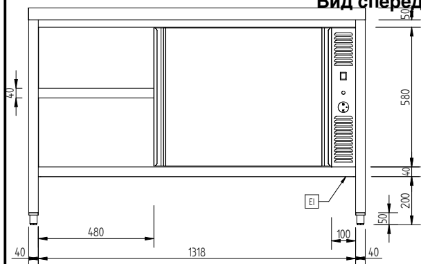
Вид спереди
