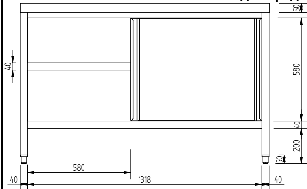
Вид сбоку
