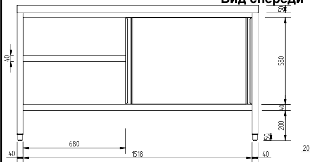
Вид спереди
