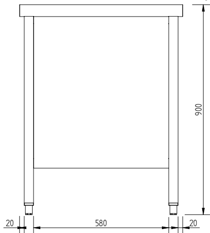
Вид сбоку
