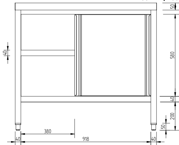
Вид спереди
