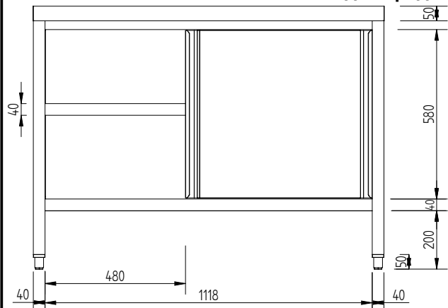
Вид спереди
