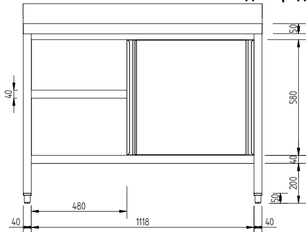
Вид спереди
