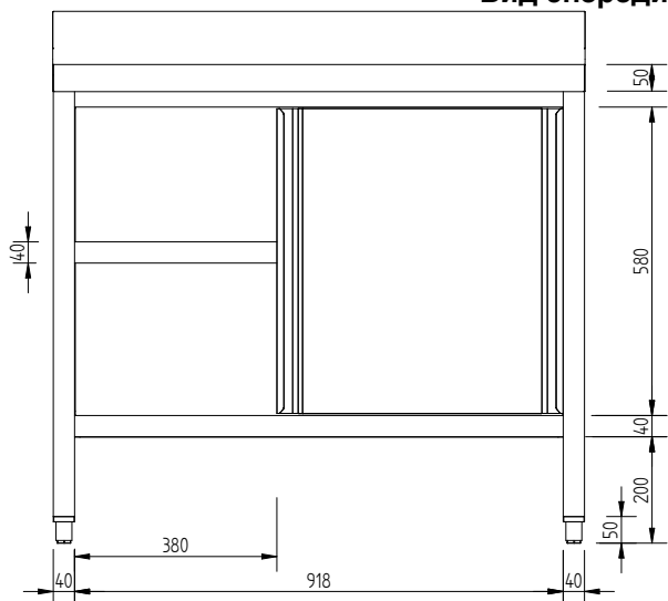
Вид спереди
