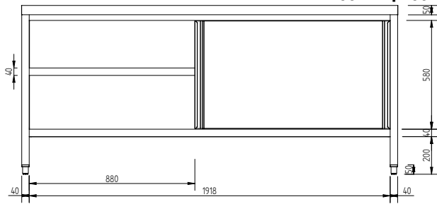
Вид сбоку
