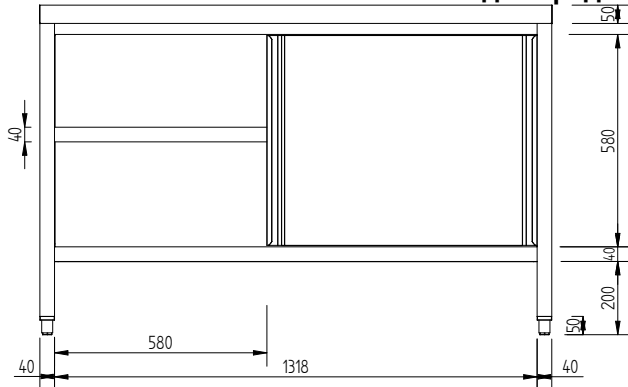
Вид спереди
