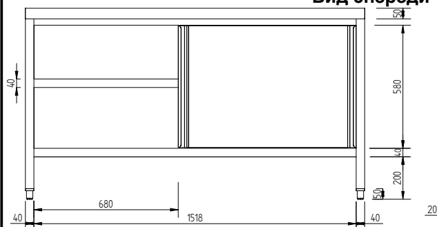
Вид спереди
