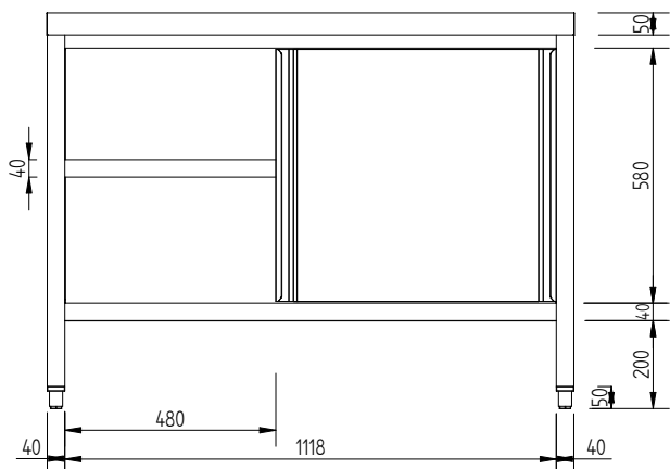
Вид спереди
