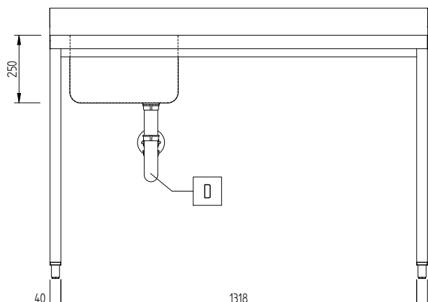
Вид сбоку
