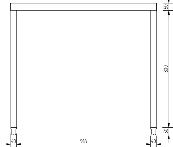
Вид спереди
