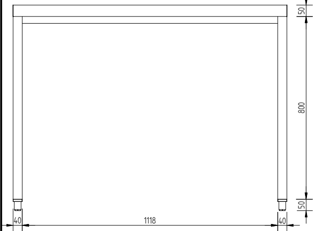
Вид спереди
