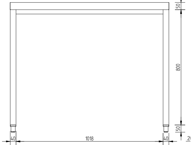
Вид спереди
