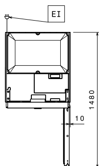
Вид сверху
