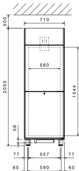
Вид спереди
